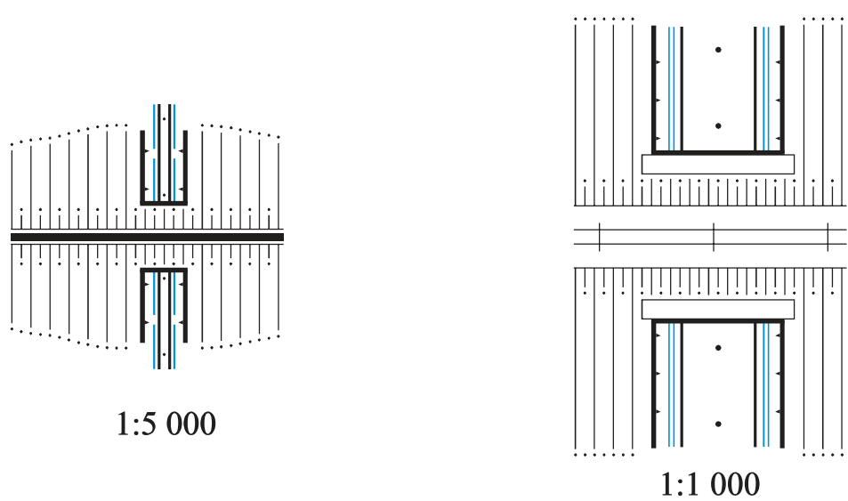
Путепроводы туннельные вне населенных пунктов
