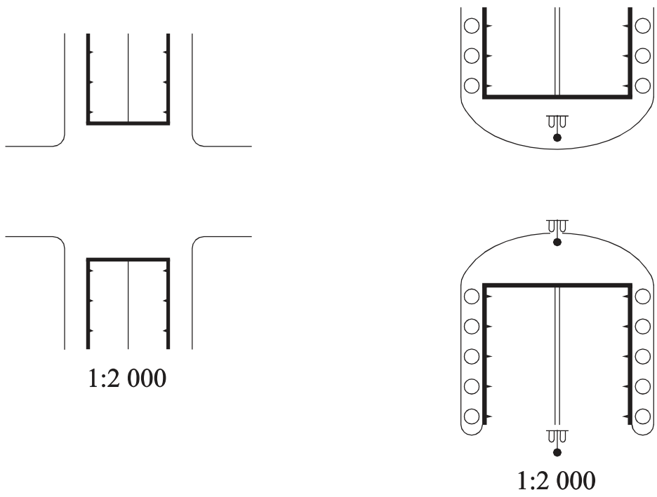
Путепроводы туннельные в городах
